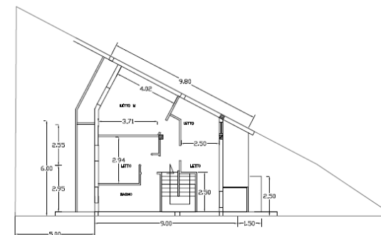
PIANO PRIMO
